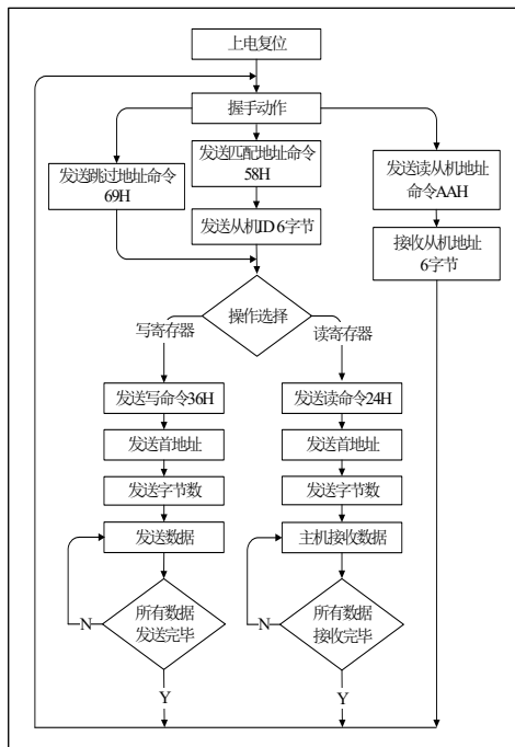
图 5. 单总线通信
