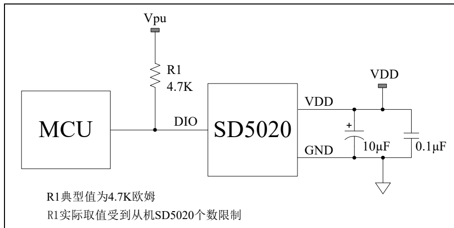
图 7. 典型应用图
