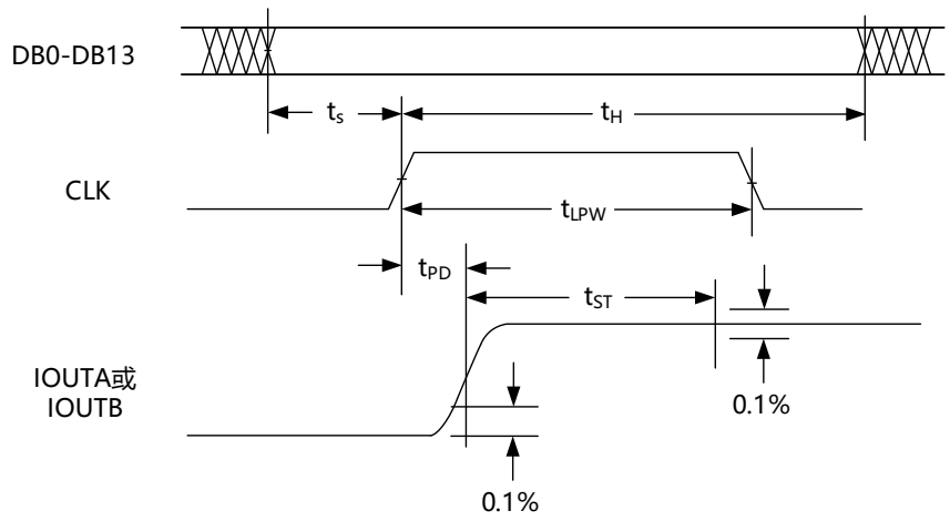
MS9734 时序图
