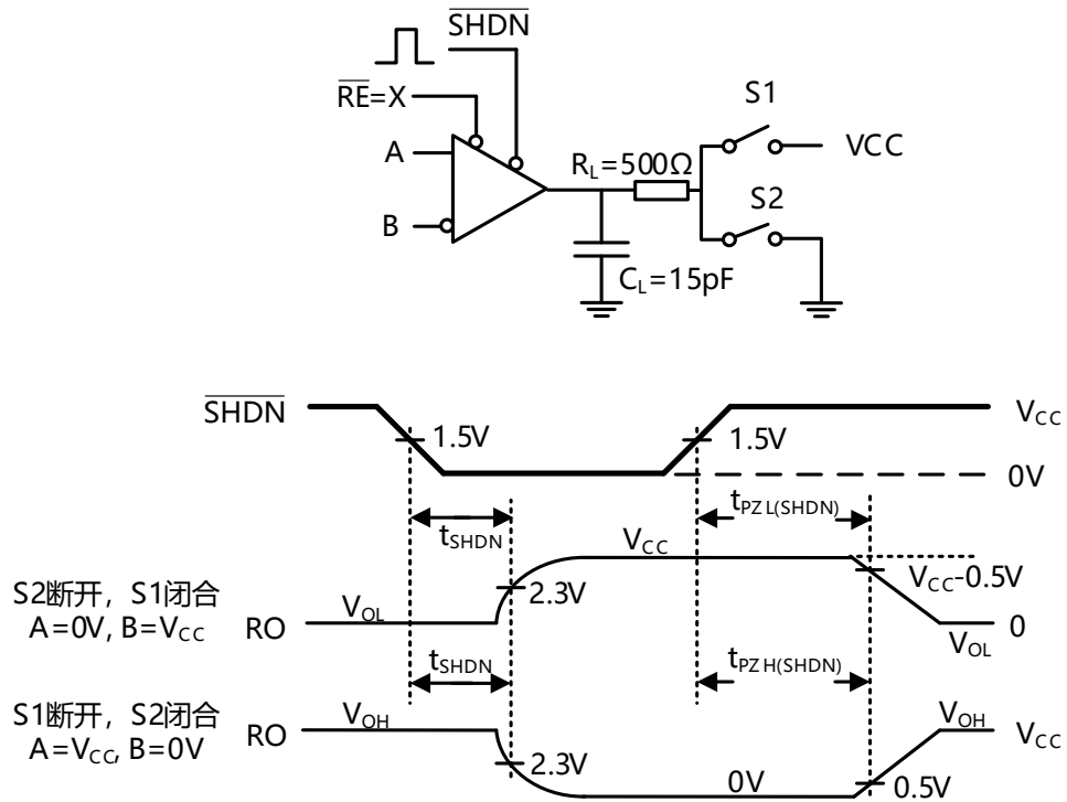
图8. 接收器开启与关断时序图 (通过SHDN开关)
