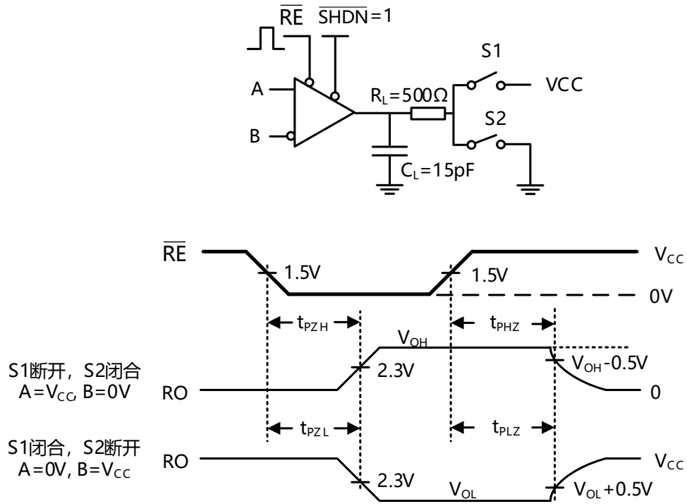
图7. 接收器开启与关断时序图 (通过RE开关)
