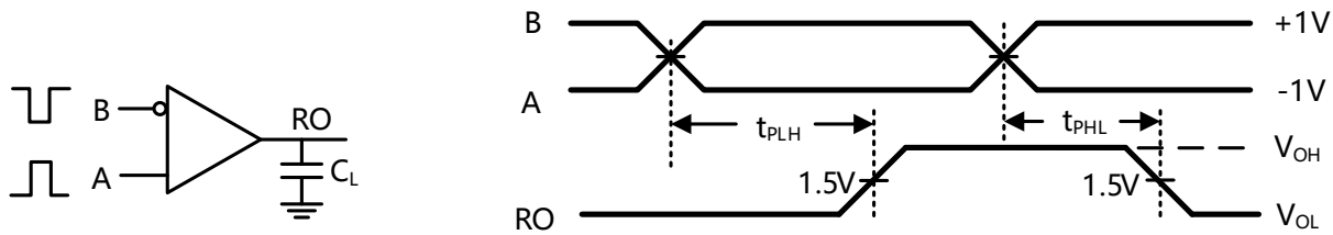
图5. 接收器传输延时测试电路
