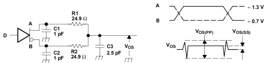
图 3. 驱动器输出共模电压的测试定义
