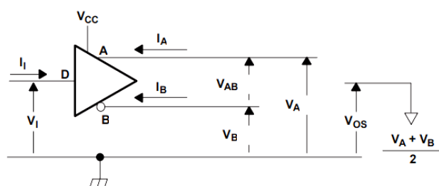
图 1. 驱动器电流和电压的定义
