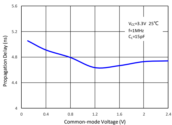
图8. 传输延时 VS. 共模电压
