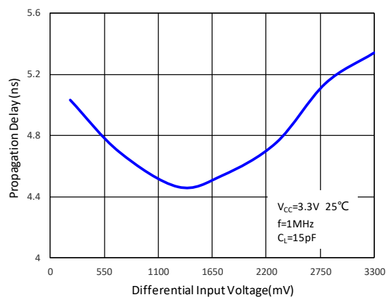
图9. 传输延时 VS. 差分输入电压
