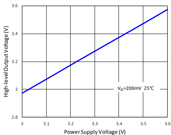
图5. 输出高电压 VS. 电源电压
