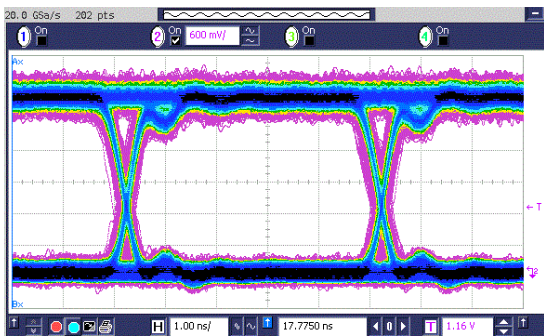
图10. 典型接收器输出眼图(200Mbps)
