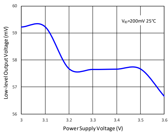
图6. 输出低电压 VS. 电源电压
