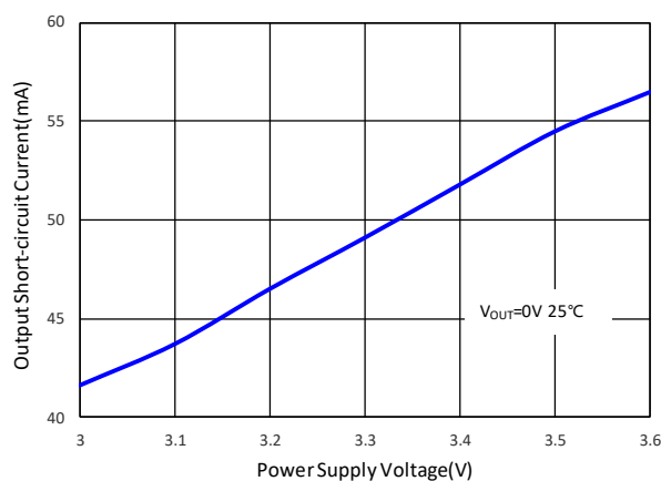
图7. 输出短路电流 VS. 电源电压
