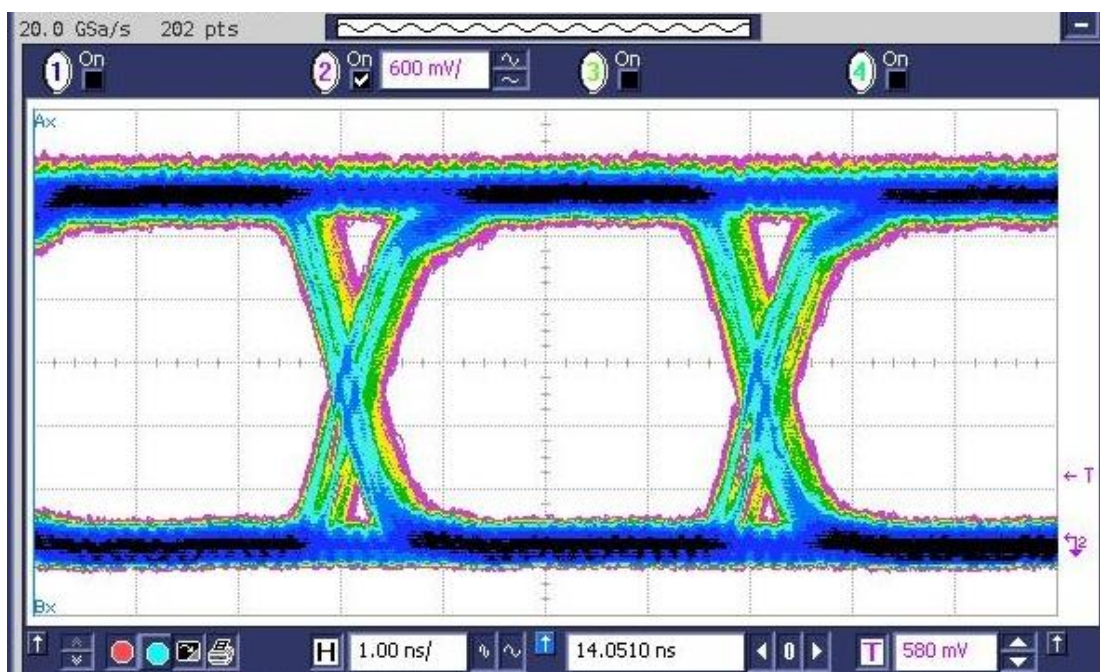
图11. 典型接收器输出眼图(250Mbps)
